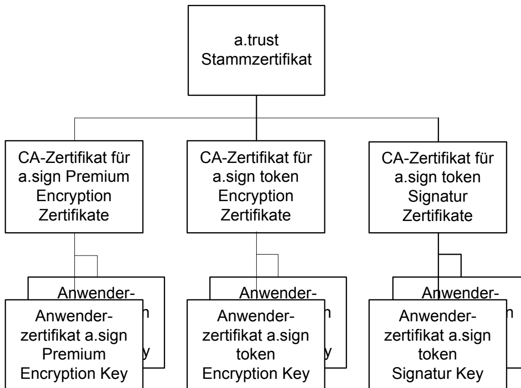
Abbildung 1 Zertifizierungshierarchie
