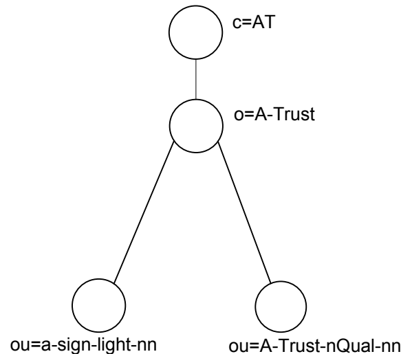
Abbildung 2 a.trust Verzeichnisbaum
